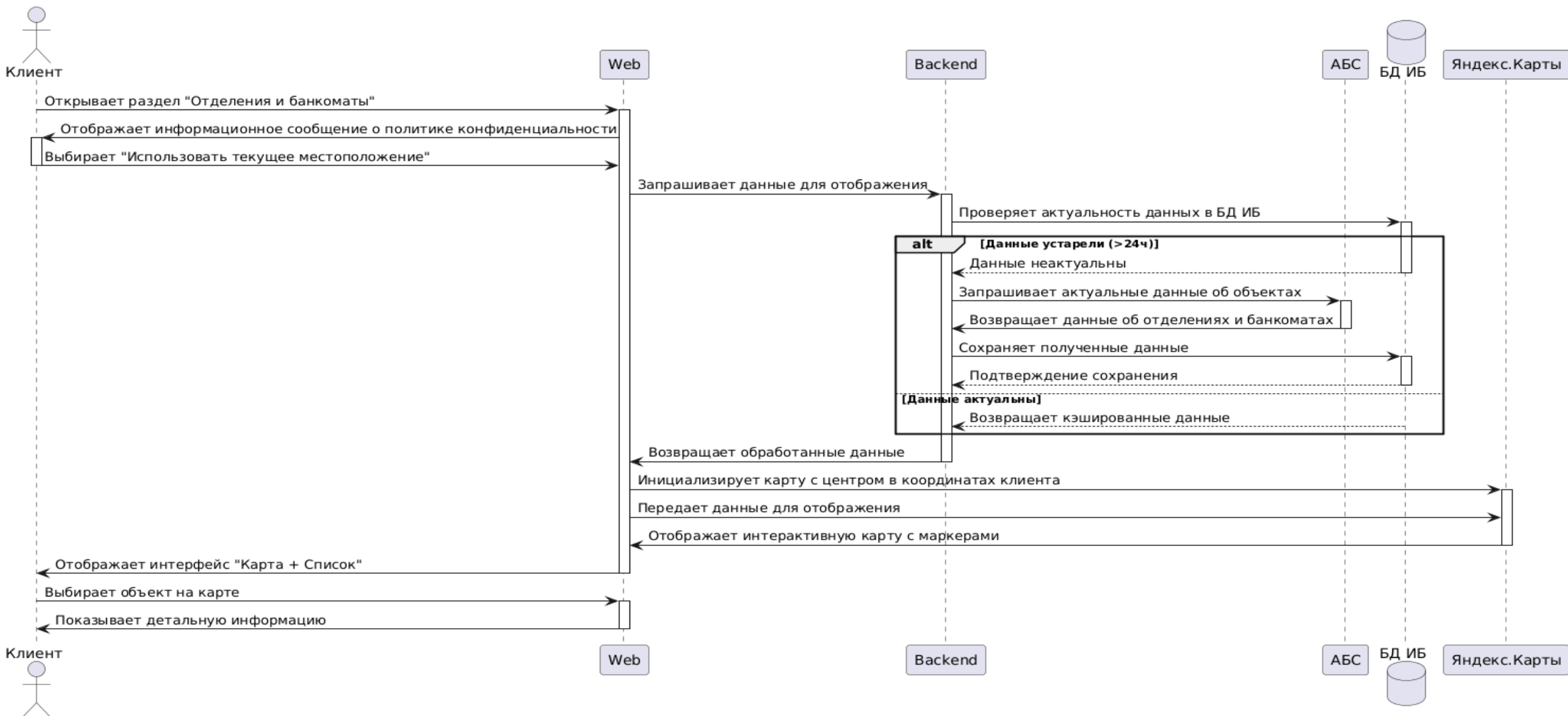
Диаграмма последовательности: Поиск ближайших объектов
